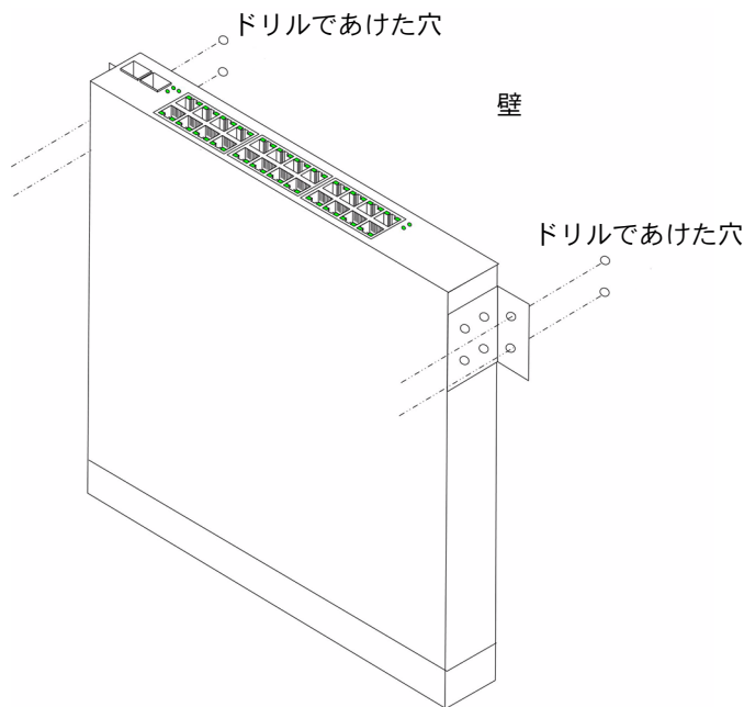
図 1-3 壁面への装置の設置
